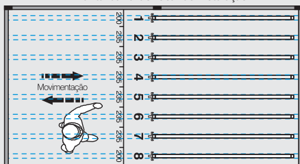
Planta-baixa do local de instalação
